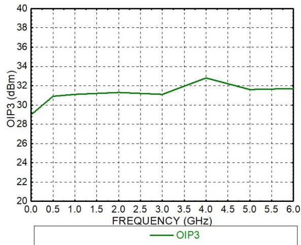
OIP3@VG接地
