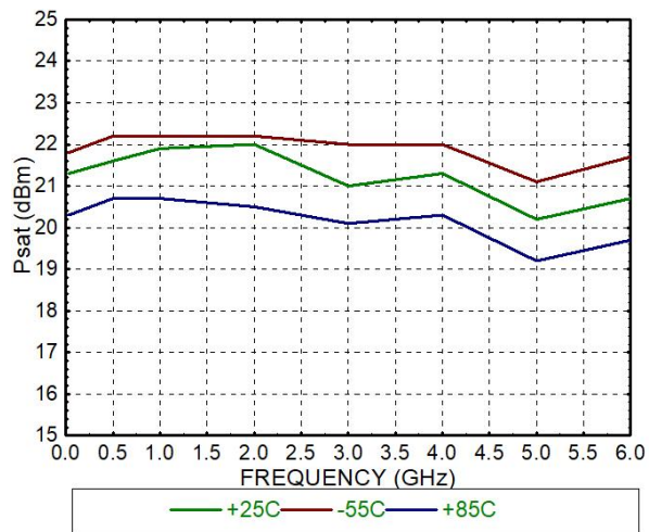
Psat@VG悬空
