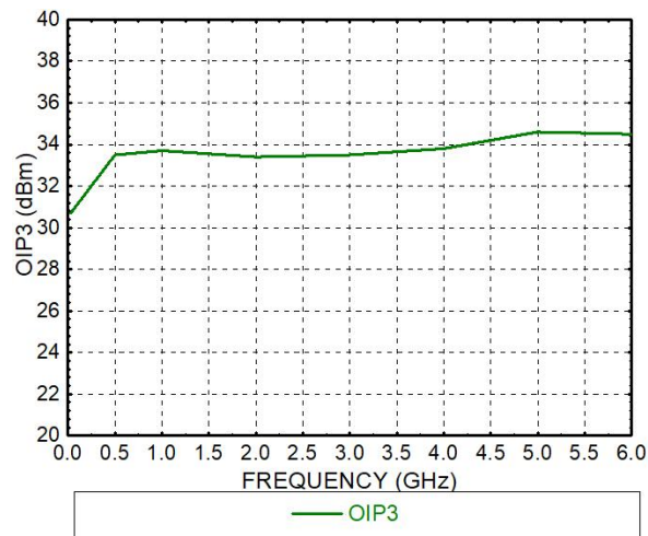
OIP3@VG悬空
