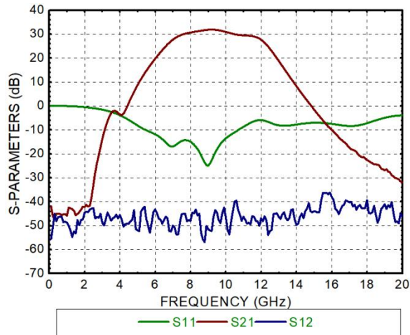
S参数
