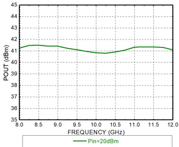
输出功率
