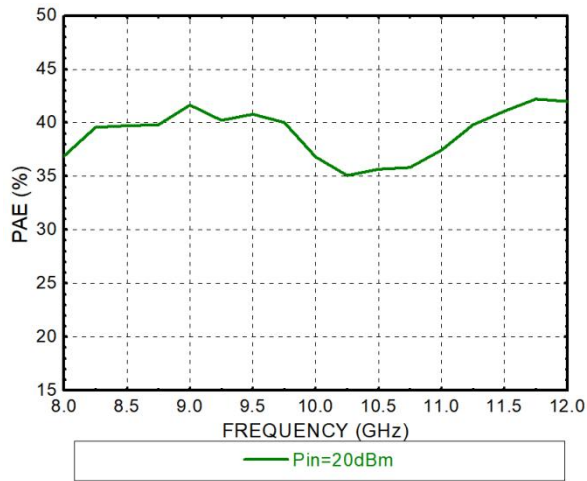
PAE
