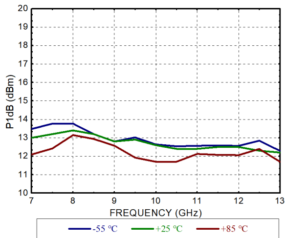
输出功率 P_{1\text{dB}} VS 温度
