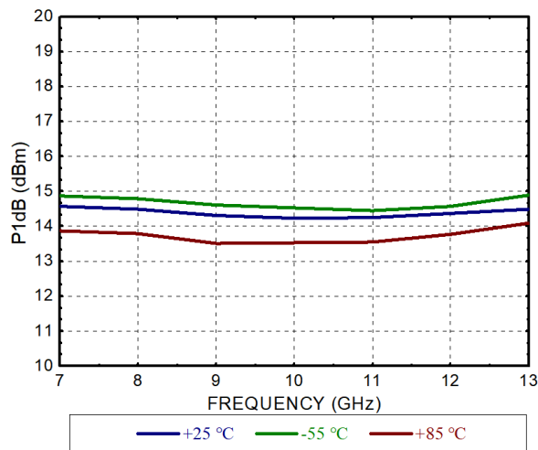
输出功率 P_{-1} VS 温度
